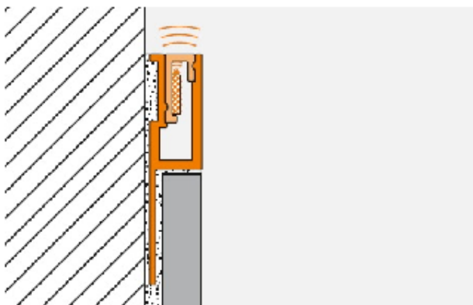
exemplo montagem luz indireta
