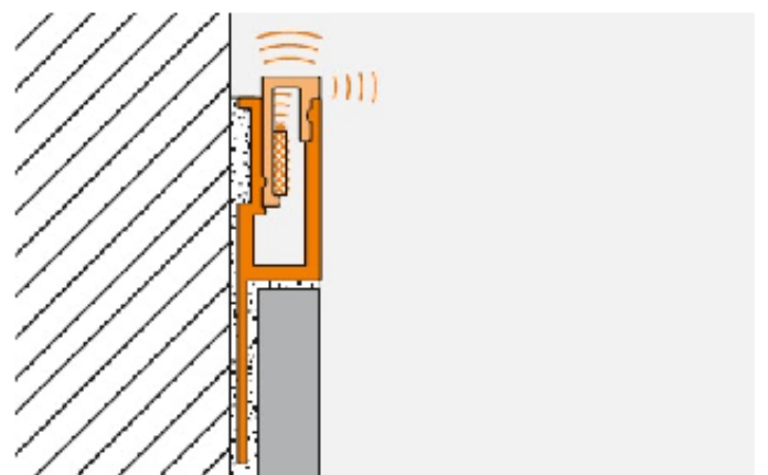
exemplo montagem luz direta e indireta
