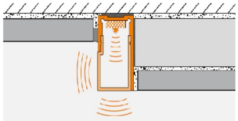
exemplo montagem luz direta
