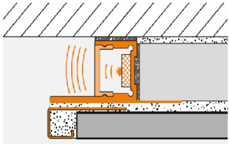
exemplo montagem luz indirecta
